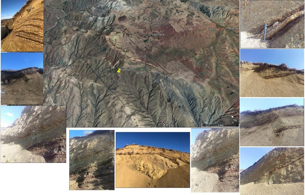
Şekil 10. Kazmaca Köyü batısında işletilmeyen kapalı kömür ocağının GoogleEarth uydu görüntüsü üzerindeki konumu ile ocak çevresinde yer alan mostralarda gözlenen kömür horizonları ile eşlik eden kırıntılı tortulların görünümü (Location of the closed coal mine not operated in the west of Kazmaca Village on the satellite image coal horizons around the coal quarry and the appearance of clastic sediments).
