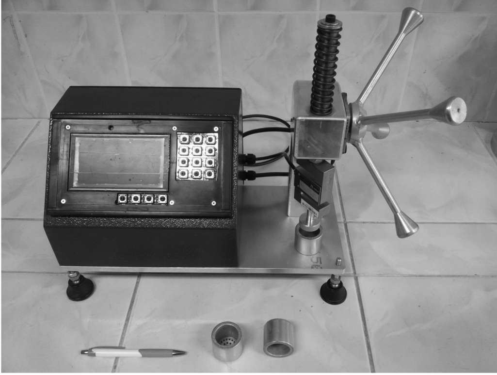
Figure 2. A view of the mud press machine and its components. Şekil 2. Çamur sıkma makinası ve bileşenlerinden bir görünüm.
