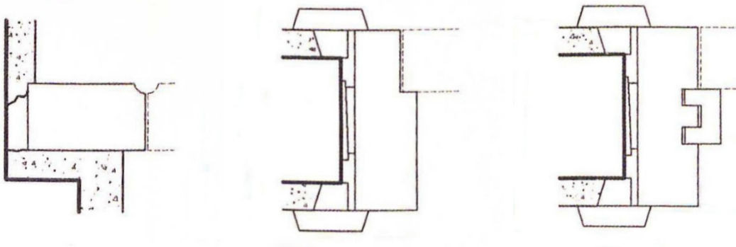
Şekil 8. Ahşap kasa çeşitleri birleşim detayları (Soldan sağa: Binisiz, tek binili, bini çıtalı ) (İzgi & Aysel, 2003)
