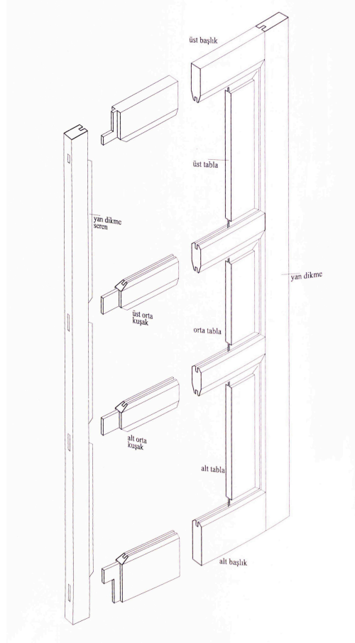
Şekil 7. Geçme tekniği detayı (İzgi & Aysel, 2003)
