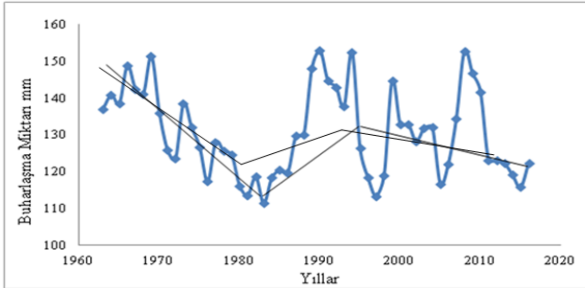
Şekil 2. Adana istasyonu buharlaşma verileri dönemsel eğilimleri Figure 2. Adana station evaporation data periodic trends
