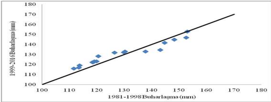
Şekil 4. Buharlaşmanın 1981-1998 ile 1999-2016 dönemlerinin grafiksel yöntem ile karşılaştırılması. Figure 4. Comparison of the evaporation period of 1981-1998 and 1999-2016 with the graphical method
