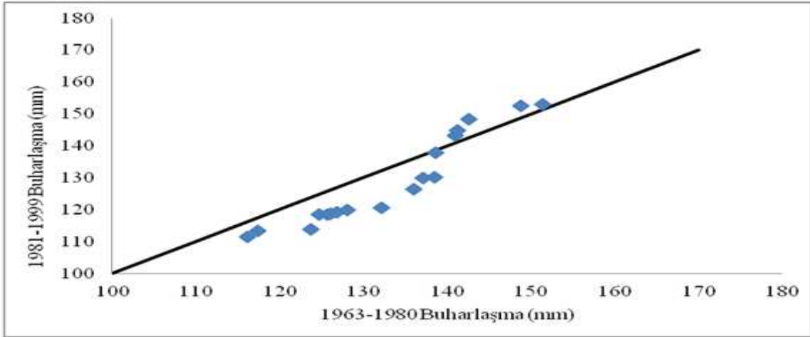
Şekil 3. Buharlaşmanın 1963-1980 ile 1981-1998 dönemlerinin grafiksel yöntem ile karşılaştırılması Figure 3. Comparison of the evaporation period of 1963-1980 and 1981-1998 with the graphical method
