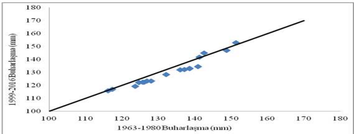
Şekil 5. Buharlaşmanın 1963-1980 ile 1999-2016 dönemlerinin grafiksel yöntem ile karşılaştırılması. Figure 5. Comparison of the evaporation period of 1963-1980 and 1999-2016 with the graphical method
