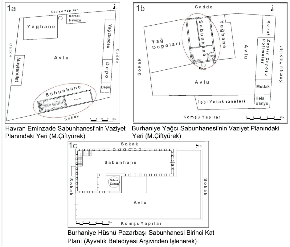
G. 23: Farklı Birimlerle Bir Avlu İçerisinde Bulunan Sabunhanelerden Örnekler (Çiftiyörek, "Türkiye'de Sabunhaneler", 342, 350, 356)
