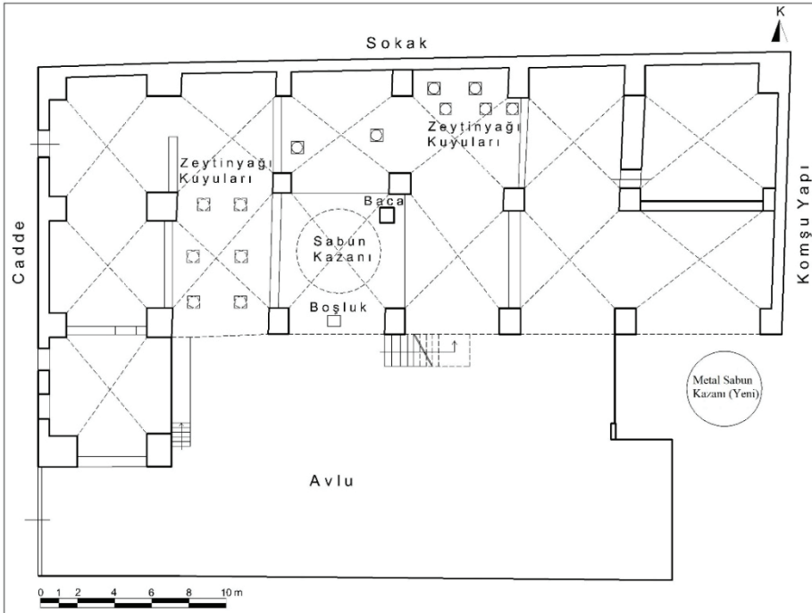
G. 8: Selahattin Ökten Sabunhanesi'nin Zemin Kat Planı (Çiftçürek, "Türkiye'de Sabunhaneler", 369)
