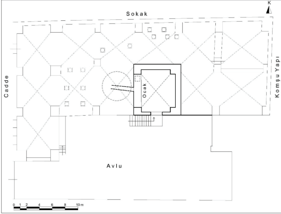
G. 15: Selahattin Ökten Sabunhanesi Ocaklık Planı (Çiftiyürek, “Türkiye’de Sabunhaneler”, 369)
