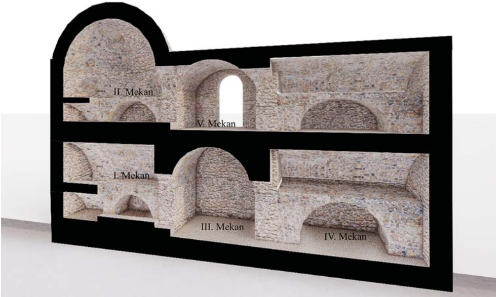
Levha 5: Anemurium A I 6 Nolu Mezar; Mekanlar ve Restitüsyon Önerisi.
