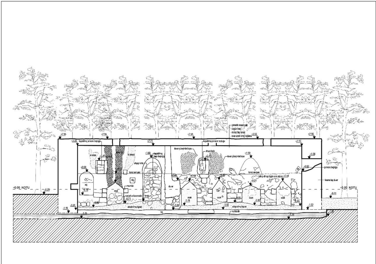
Şekil 5. Aynül Meydan Çamaşırhanesi A-A kesiti röleve çizimi / A-A section survey drawing of Aynül Meydan Laundry (Doğru, 2019).
