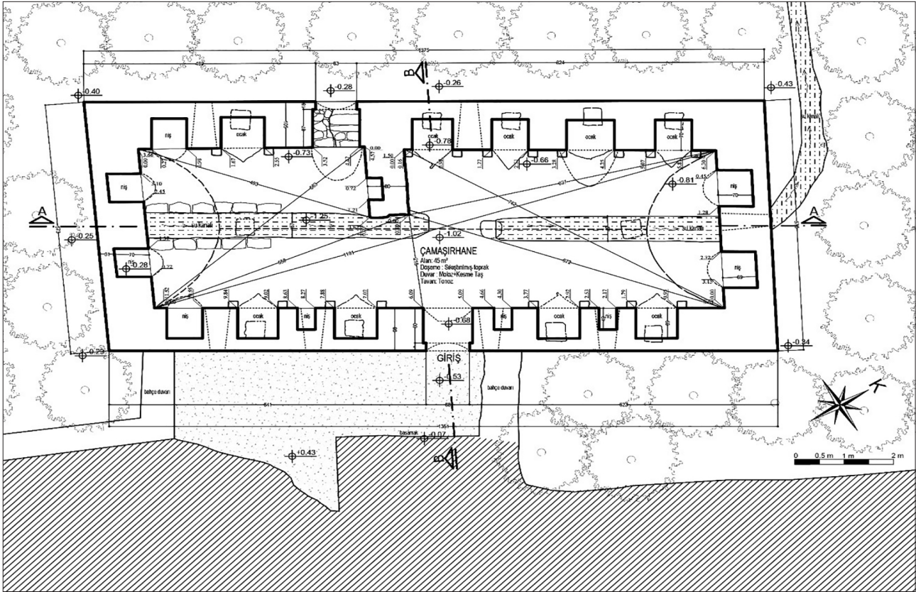
Şekil 4. Aynül Meydan Çamaşırhanesi röleve planı / The survey plan of Aynül Meydan Laundry (Doğru, 2019).
