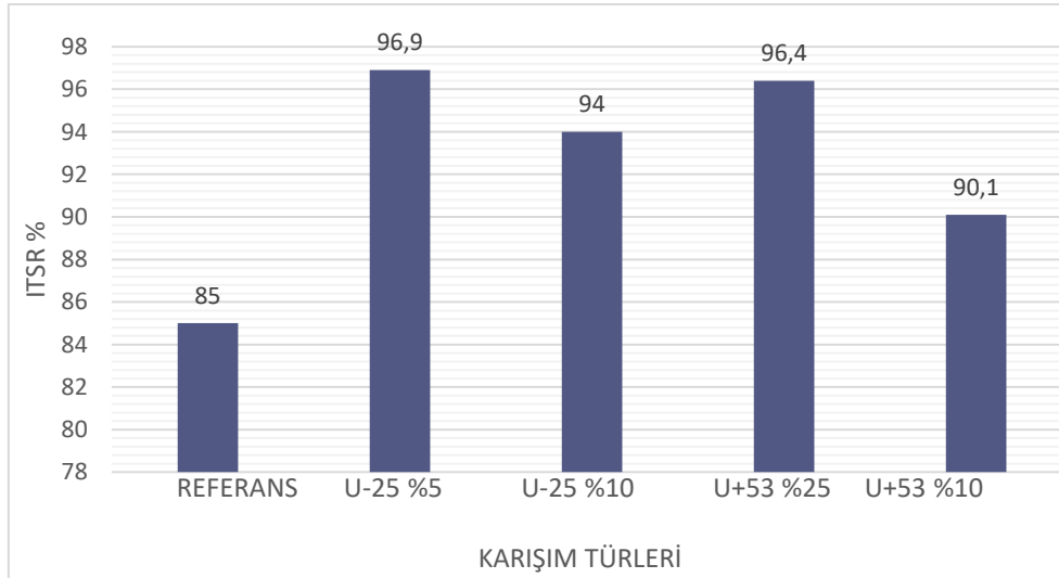
Şekil 11. U-25 ve U+53 üleksit mineralleriyle hazırlanan asfalt karışımların dolaylı çekme mukavemeti oranları değişimleri
