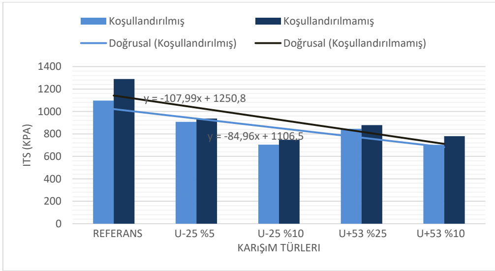
Şekil 10. U-25 ve U+53 üleksit mineralleriyle hazırlanan asfalt karışımların ITS değeri değişimleri
