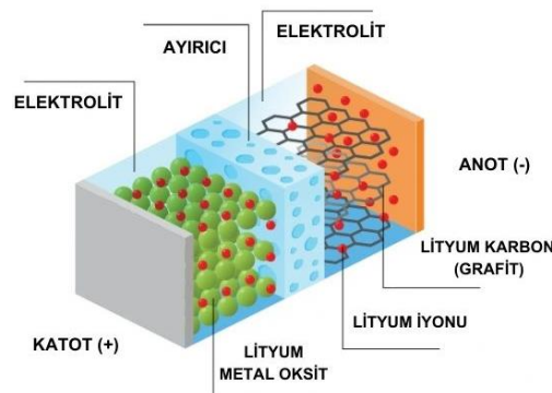
Şekil 2. Bir LIB'nin yapısı [9] (Structure of a LIB)
