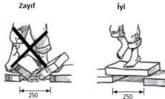
Şekil 6. Kerpiç blok basınç dayanımı saha deneyi (TSE, 1977).
