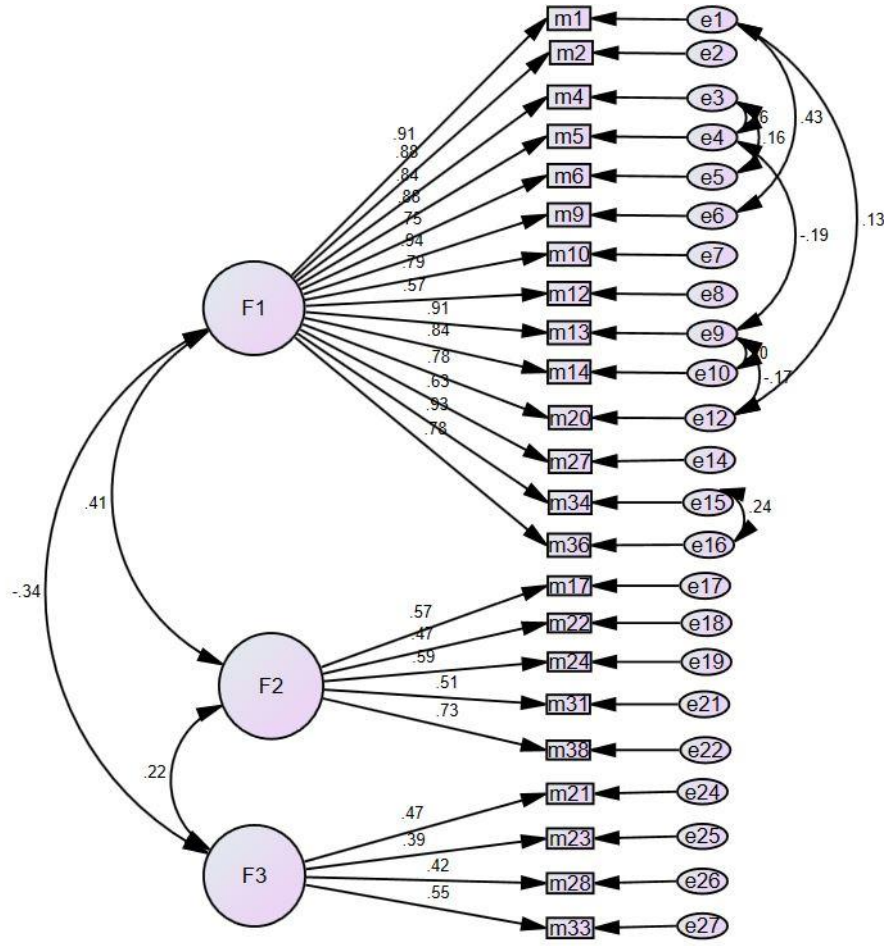
Şekil-1: İslam Din Okuryazarlığı Ölçeğine Ait Path Diyagramı
