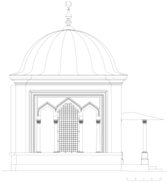
Çizim 3. Yan Cephe
