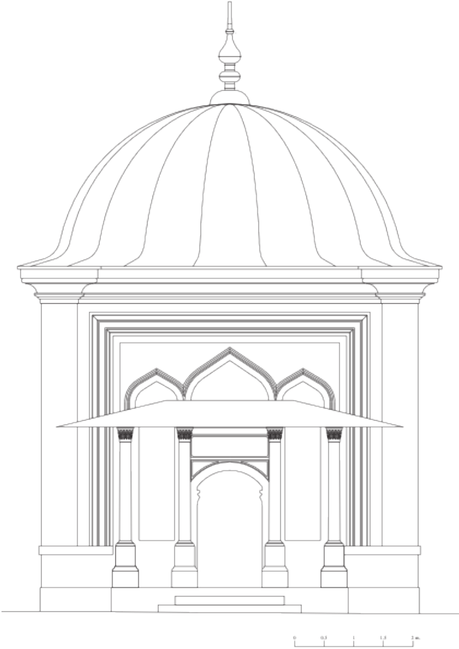
Çizim 2. Ön Cephe
