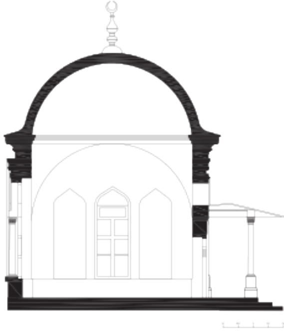
Çizim 5. Kesit
