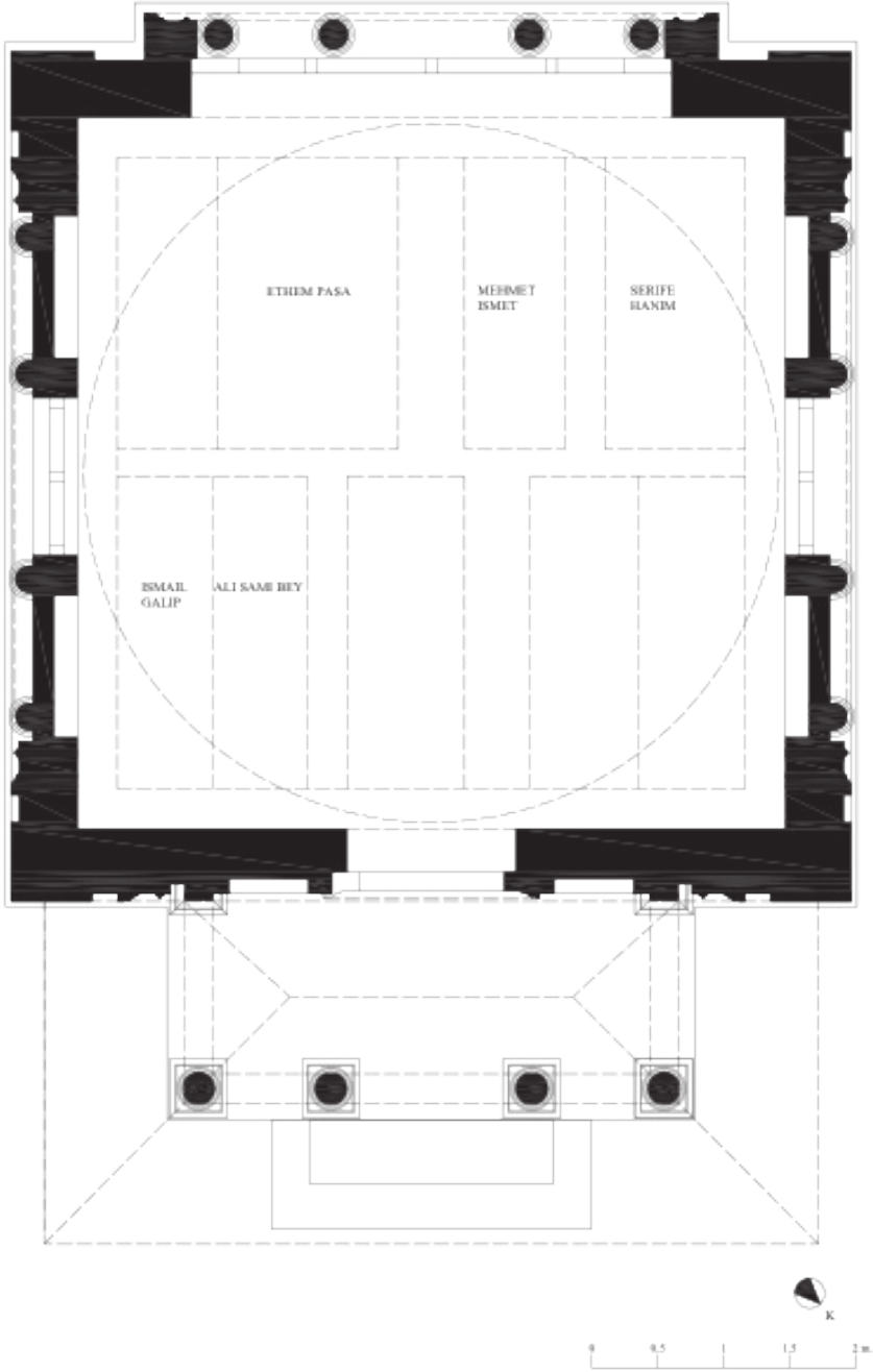
Çizim 1. İbrahim Edhem Paşa Türbesi Plan
