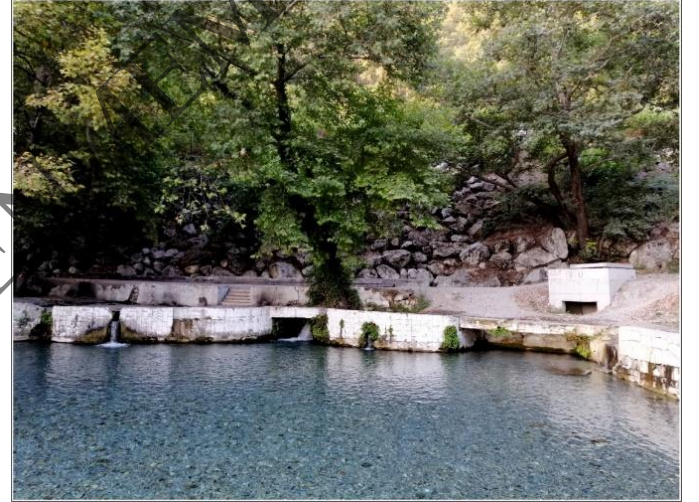
Şekil 23. Pınarbaşı Kaynağı. Honaz fayının batı ucuna yakın (Şekil 21) bir noktada yer alır (foto: Mehmet Özkul).
