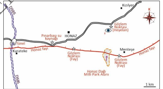
Şekil 21. Honaz Fayı üzerindeki gözlem (temas) noktaları. Figure 21. Points of interest on the Honaz Fault.
