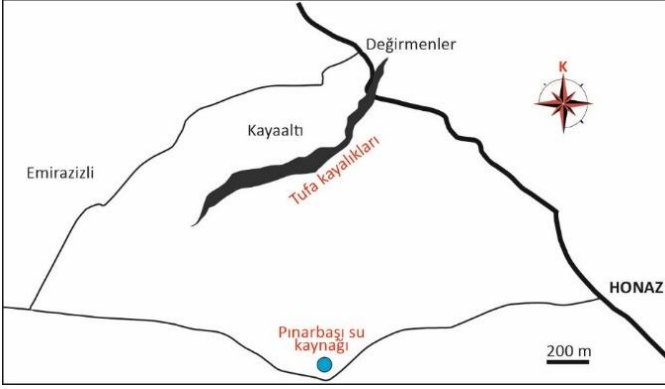
Şekil 24. Pınarbaşı kaynağı, Kayalı tufa kayalıkları ve Değirmenler temas noktalarının konumu.
