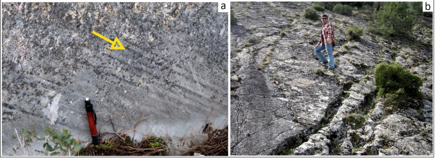
Şekil 22. Menteşe Mahallesi yakınındaki ilgi noktasında (Şekil 21) Honaz fay düzleminde görüntüler. (a) Kayma çizikleri (okla işaretli), (b) Fay düzleminde oluk yapısı (fotolar: Mete Hançer).
