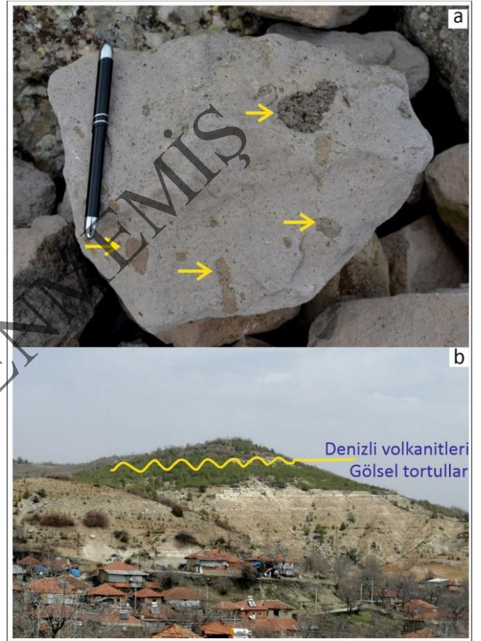
Şekil 12. Denizli volkanitleri. (a) Volkanitlerde 'cognate' anklavlar (oklar). Anklavların çevresine göre daha koyu renkli olduklarına dikkat ediniz, (b) Üst Miyosen-Pliyosen gölsel istifi üzerine uyumsuz olarak gelen Denizli volkanitleri, Kocapınar Mahallesi, Serinhisar (fotolar: Barış Semiz).
