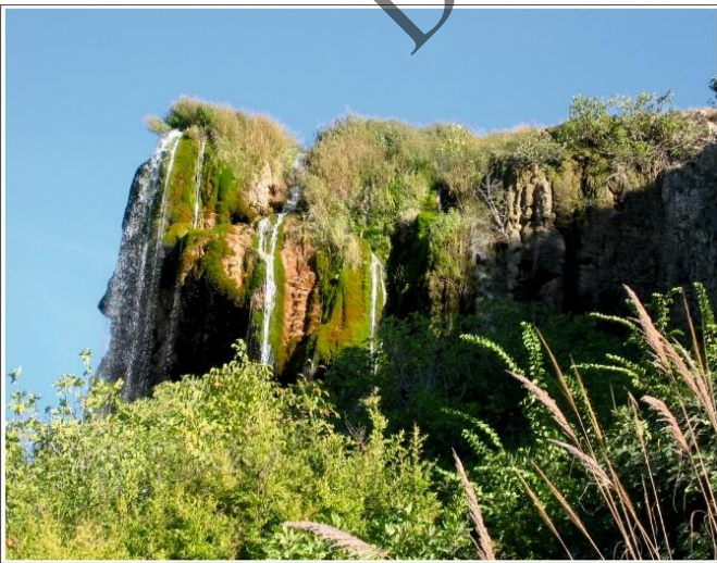
Şekil 18. Güney şelalesi jeositinden bir görünüm (foto: Mehmet Özkul).
