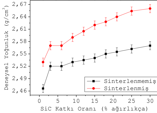
Şekil 5. Al-SiC kompozit yapılarında SiC katkı oranıyla deneysel yoğunluğun değişimi (Figure 5. The variation of experimental density with SiC content in Al-SiC composites)
