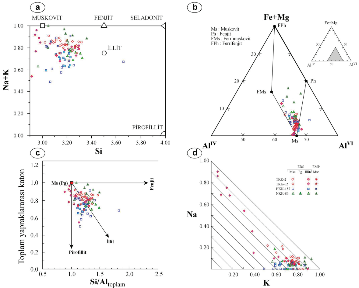
Şekil 9. Karakaya Karmaşığı birimlerine ait istif içeren kumtaşı/metakumtaşılarındaki illit/muskovit minerallerinin bileşimlerdeki katyonlara göre ikili ve üçgen diyagramlarda konumları, a) Yapraklararası Na+K–tetrahedral Si, b) Oktahedral (Fe+Mg)–oktahedral Al IV –tetrahedral Al VI , c) Yapraklararası katyonlar toplam –tetrahedral Si/Al toplam , d) Yapraklararası Na–K.
