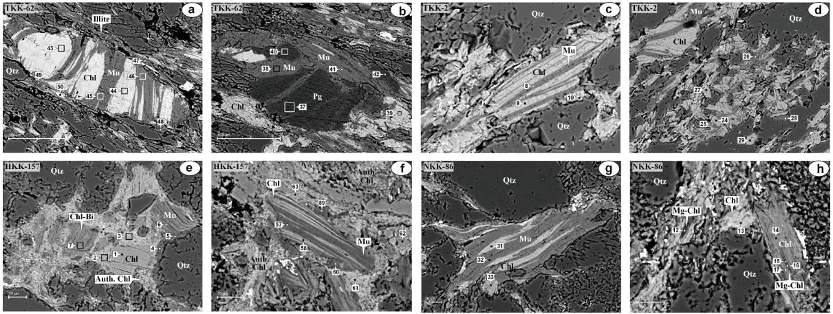
Şekil 5. Karakaya Karmaşığı birimlerine ait istif içeren metakumtaşlarının BSE mikrofotografaları (TKK-62 ve TKK-2: Turhal Metamorfitle, HKK-157: Hodul Birimi, NKK-86: Orhanlar Birimi, Rakamlar: EDS analiz yapılan noktalar, Chl=Klorit, Mu=Muskovit, Bi=Biyotit, Ill=İllit, Pg=Paragonit, Qtz=Kuvars, Auth-Chl=Otijenik klorit), a) Klorit-muskovit istifi ve illit levhaları, b) Muskovit-paragonit istifi ve klorit levhaları, c-d) Klorit-muskovit istifi ve klorit levhaları, e-f) Klorit-biyotit istifi, klorit ve muskovit levhaları, otijenik klorit, g) Klorit-muskovit istifi, h) Klorit ve Mg-klorit levhaları.
