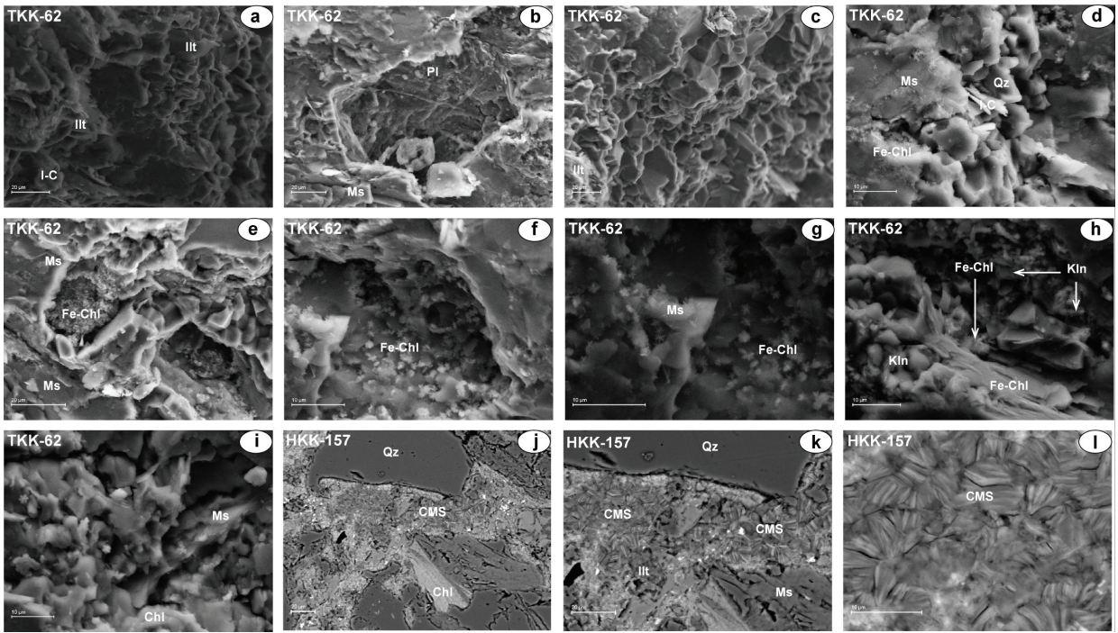
Şekil 4. Karakaya Karmaşıđı birimlerine ait istif içeren metakumtaşının SEM mikrofotografı (TKK-62: Turhal Metamorfitleri, HKK-157: Hodul Birimi, CMS=Klorit-Mika istifli, Chl=Klorit, Ms=Muskovit, Illt=İllit, Kln=Kaolinit, I-C=Karışık tabakalı illit-klorit, Qz=Kuvars, Pl=Plajiyoklaz), a) Gözenekte peteksi-yapraksı görünümlü illit ve yapraksı I-C mineralleri, b) Trigonal kuvars, yapraksı muskovitler ve gözenekte Si-Al tüpleri, c) Peteksi-yapraksı illitler, d) Yapraksı muskovit, çubuksu I-C ve tüysü-lifsi Fe-kloritler, e-f) İri yapraksı muskovitler arasındaki boşluklarda Fe-kloritler, g) Muskovit yaprakları ve Fe-klorit lifleri, h) Lifsi-çubuksu Fe-kloritler ve yapraksı kaolinitler, i) Yapraksı muskovitler ve lifsi kloritler, j)-k) Matrikste iri taneli klorit-mika istifleri ve gözeneklerde kloritler, l) Gözeneklerde ince taneli otjenik kloritlerin büyütülmüş görünümü.
