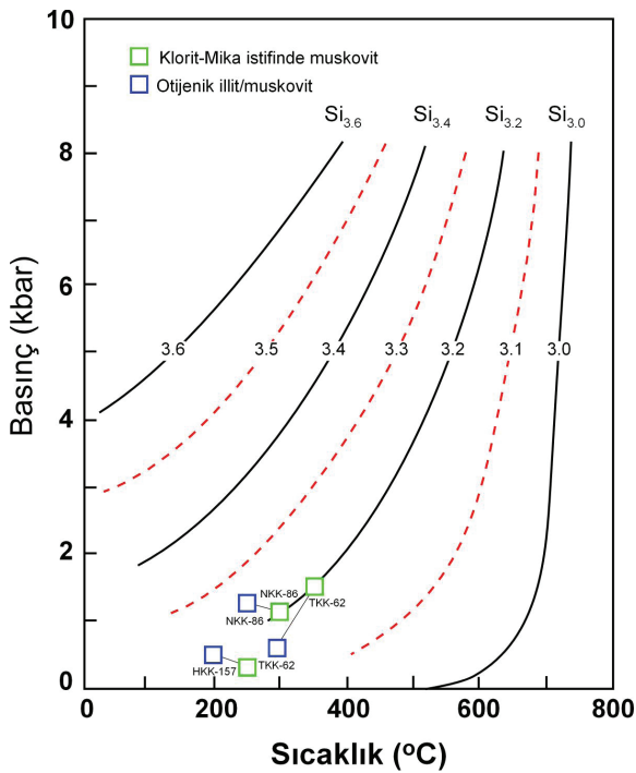
Şekil 10. Karakaya Karmaşığı birimlerine ait istif içeren kumtaşı/metakumtaşlarındaki illit/muskovit minerallerinde tetrahedral Si içeriğine göre basınç-sıcaklık diyagramı (Velde, 1967).
