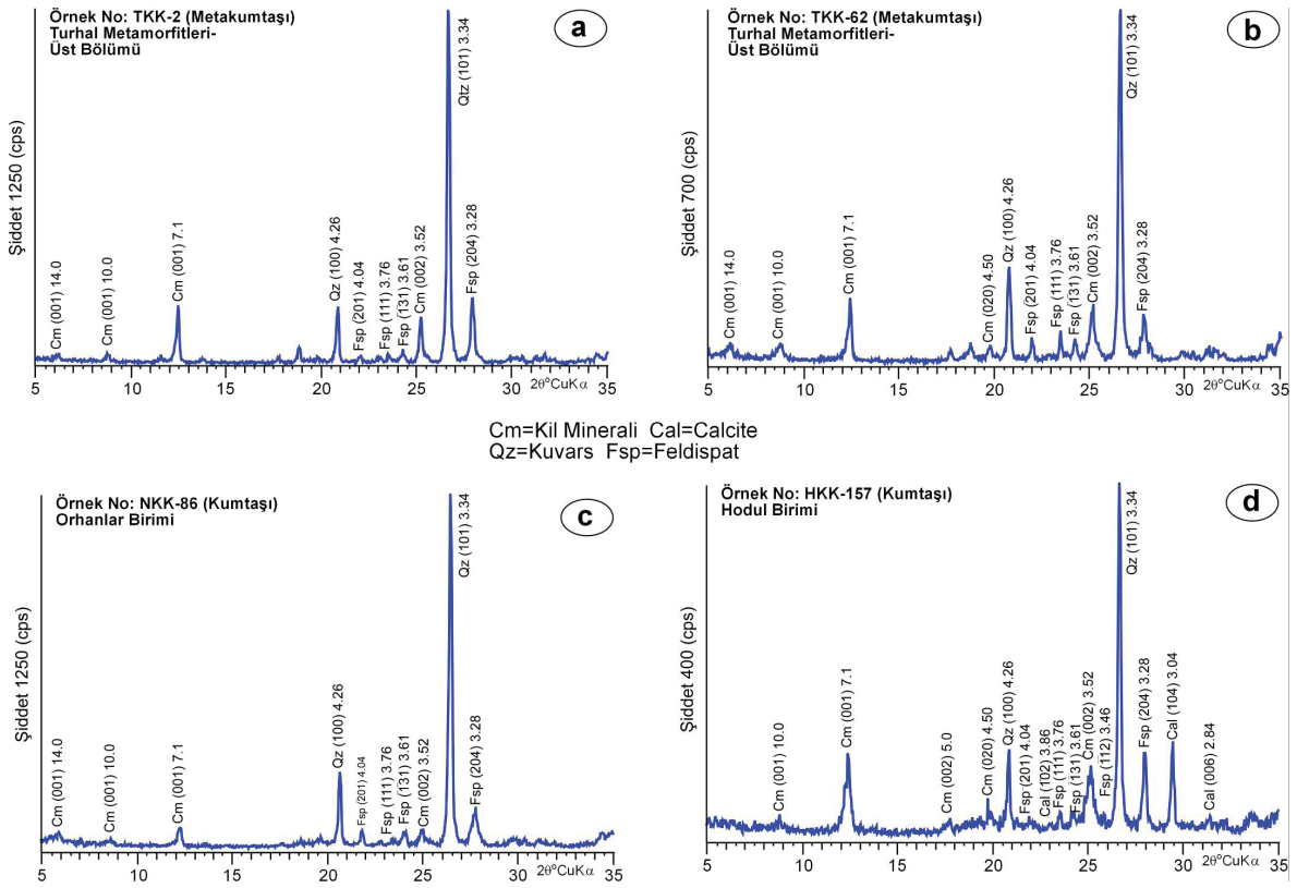
Şekil 6. Karakaya Karmaşığı birimlerine ait istif içeren kumtaşı/metakumtaşlarının XRD-TK difraktogramları, a-b) Turhal Metamorfileri, c) Orhanlar Birimi, d) Hodul Birimi,
