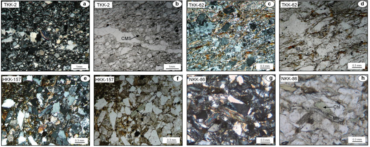
Şekil 3. Karakaya Karmaşığı birimlerine ait istif içeren kumtaşı/metakumtaşlarının optik mikroskopik mikrofotoğrafları (CMS=Klorit-muskovit istif, Chl=Klorit, M=Muskovit), a-b-c-d) Turhal Metamorfite, e-f) Hodul Birimi, g-h) Orhanlar Birimi.
