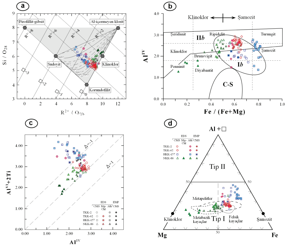
Şekil 8. Karakaya Karmaşığı birimlerine ait istif içeren kumtaşı/metakumtaşlarındaki klorit minerallerinin bileşimlerindeki katyonlara göre ikili ve üçgen diyagramlardaki konumları, a) Si/O_{28}-R^{2+}/O_{28} (Sınıflandırma: Wiewióra ve Weiss, 1990; sıcaklık eğrileri: Bourdelle ve Cathelineau, 2015), b) Tetrahedral Si-oktahedral Fe/(Fe+Mg) (Sınıflandırma ve I/b politypi alanı: Foster, 1962; I/b politypi alanı: Curtis vd. 1985; şamozit-klinoklor sınırı: Bailey, 1980), c) Oktahedral Al+2Ti -tetrahedral Al (Diyagram: Zane vd. 1998), d) Oktahedral Al+□-Mg-Fe ( □ =Oktahedral boşluk; Diyagram: Zane ve Weiss, 1998; metapelit, metabazik ve felsik kayaç alanları: Zane vd. 1998).
