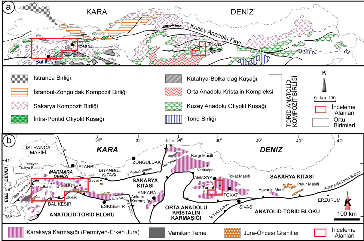
Şekil 1. a) İncelenen alanlarının Türkiye'nin Alpin Birlikleri içindeki yeri (Göncüoğlu vd. 1997), b) Karakaya Karmaşığı ve ilgili birimlerin dağılımını gösteren Kuzey Anadolu'nun tektonik haritası (Okay ve Göncüoğlu, 2004).
