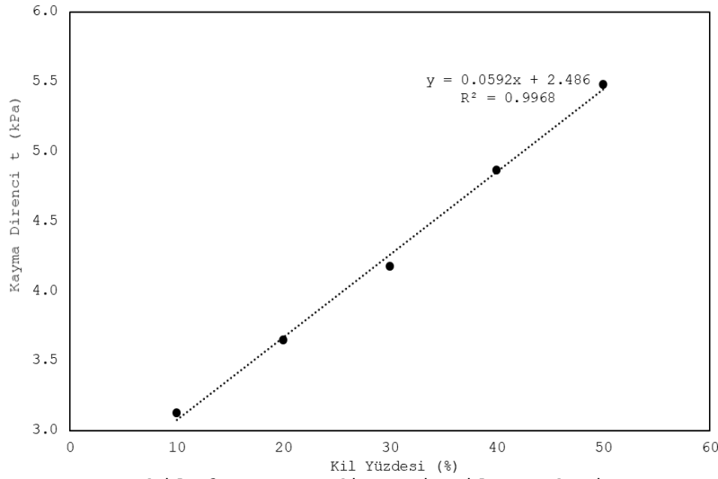
Şekil 6. Kayma direnci-Kil yüzdesi (Figure 6. Shear strength-Clay percentage)
