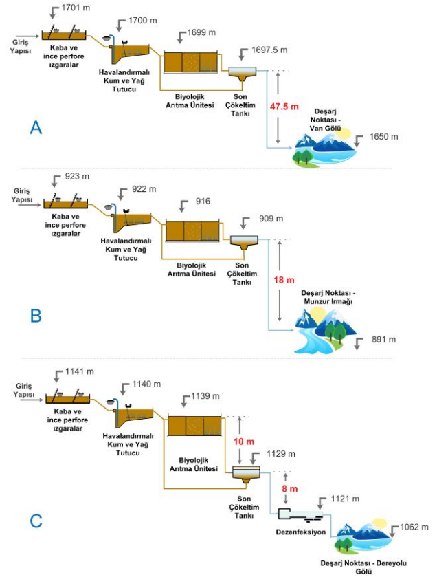
Şekil 4. Her üç tesise ait akım şemaları ve rakım bilgileri (A: Van-Edremit AAT, B: Tunceli AAT ve C: Elazığ-Sivrice AAT).
