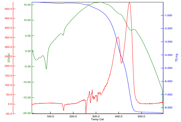
Şekil 13. BS3 besleme stoku Termal Analiz eğrileri
