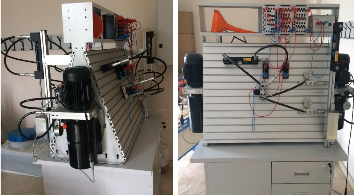
Şekil 1. Karşılaştırma deneyleri için kullanılan deney düzeneği
