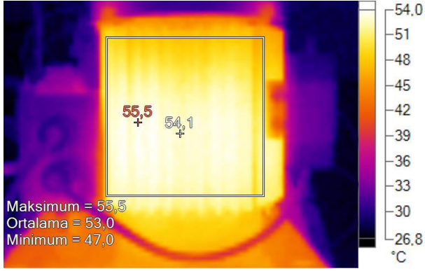
Şekil 4. Sıvı deneyi için elektrik motorunun termal ve normal görüntüsü
