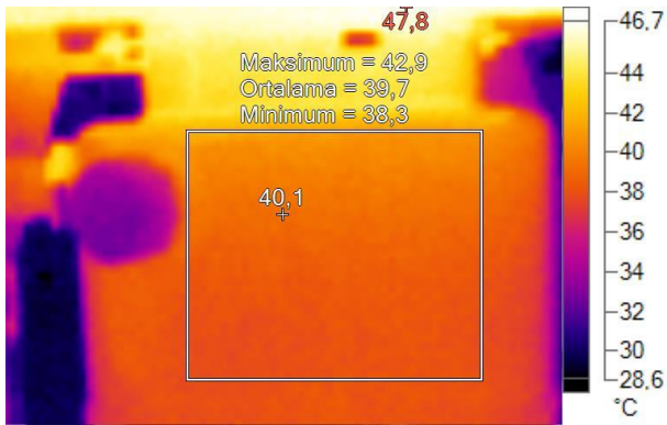
Şekil 6. Sıvı için yürütülen deneyde tankın termal ve normal görüntüsü
