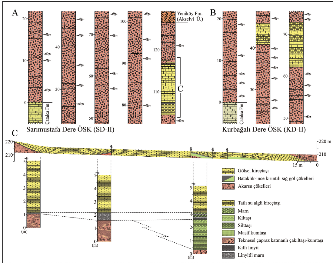
Şekil 7. Bahçecik formasyonundan alınan ölçülü stratigrafi kesitleri. A) Sarımustafa Dere ÖSK (SD-II), B) Kurbağalı Dere ÖSK (KD-II). Kesit güzergahları Şekil 6-A'da gösterilmiştir.
