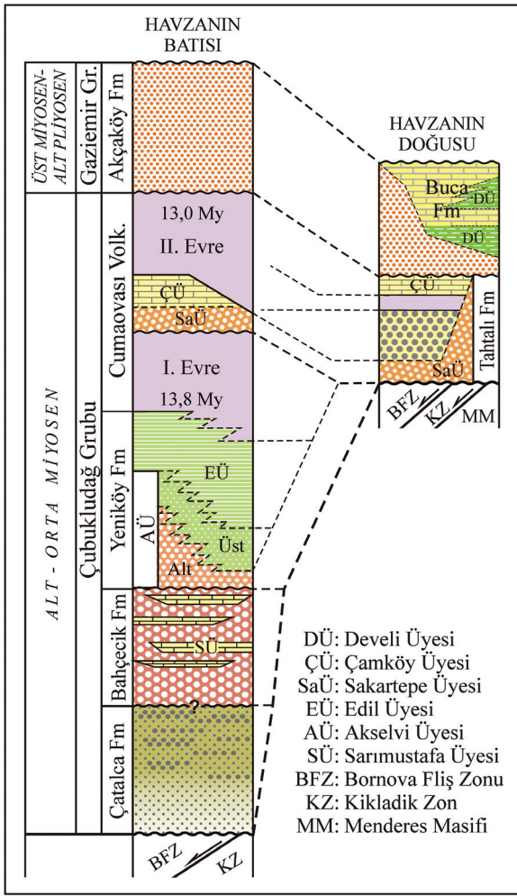
Şekil 3. Çubukludağ havza dolgusunun genelleştirilmiş stratigrafi kesiti.
