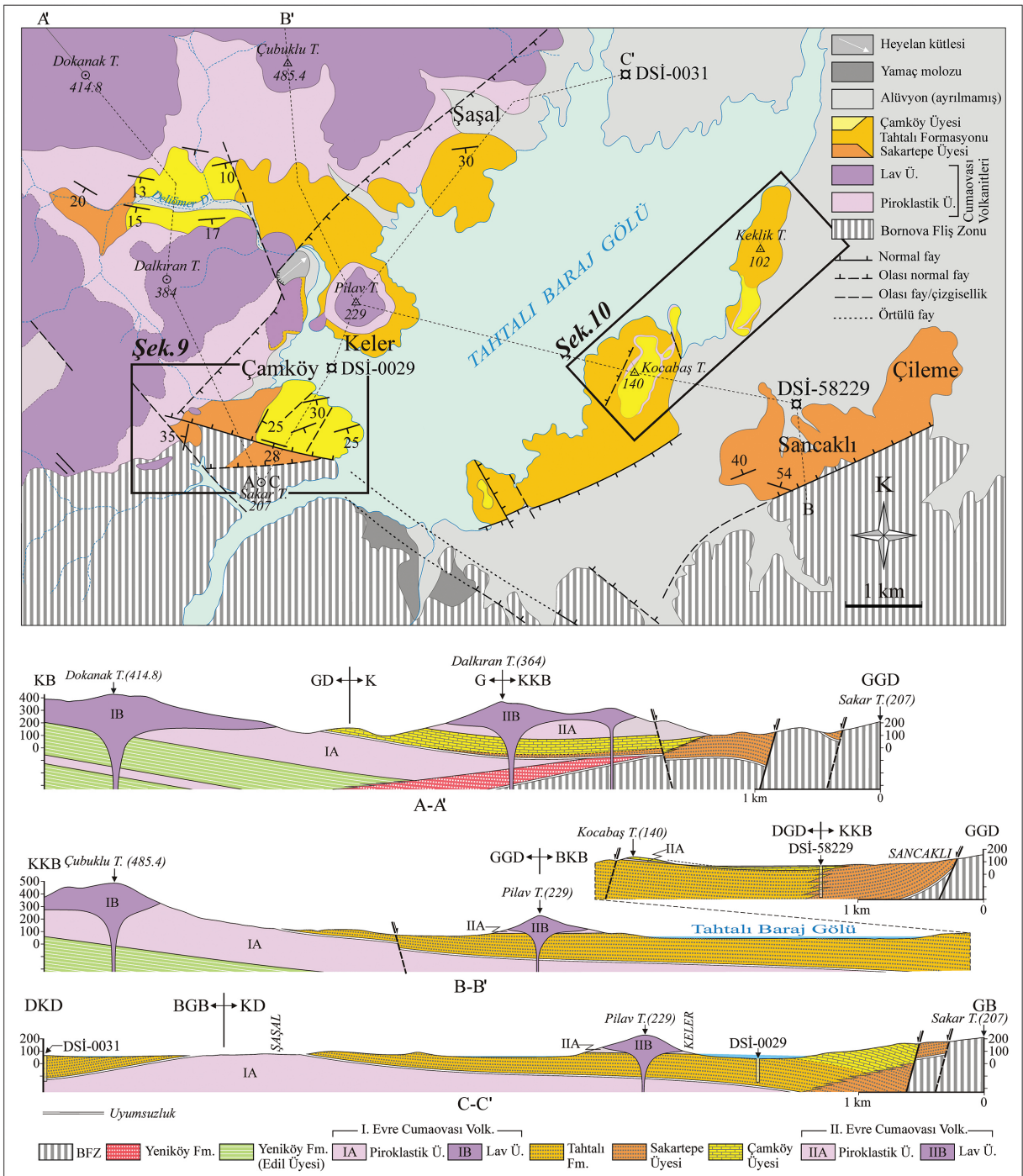
Şekil 8. Tahtalı Baraj Gölü çevresinde yüzeyleyen Tahtalı formasyonunun jeoloji haritası ve jeoloji enine kesitleri. Figure 8. Geological map and cross sections of Tahtalı formation exposed in the vicinity of Tahtalı Dam Lake.
