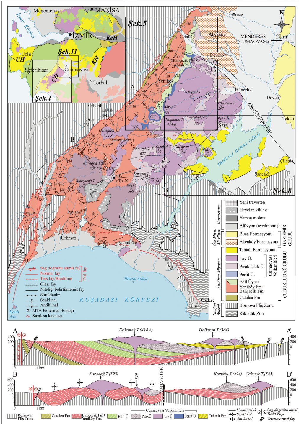
Şekil 4. Çubukludağ havzasının jeoloji haritası (Eşder, 1988'den değişiklikle). UH: Urla Havzası, ÇH: Çubukludağ Havzası, KH: Kocaçay Havzası, KeH: Kemalpaşa Havzası.
