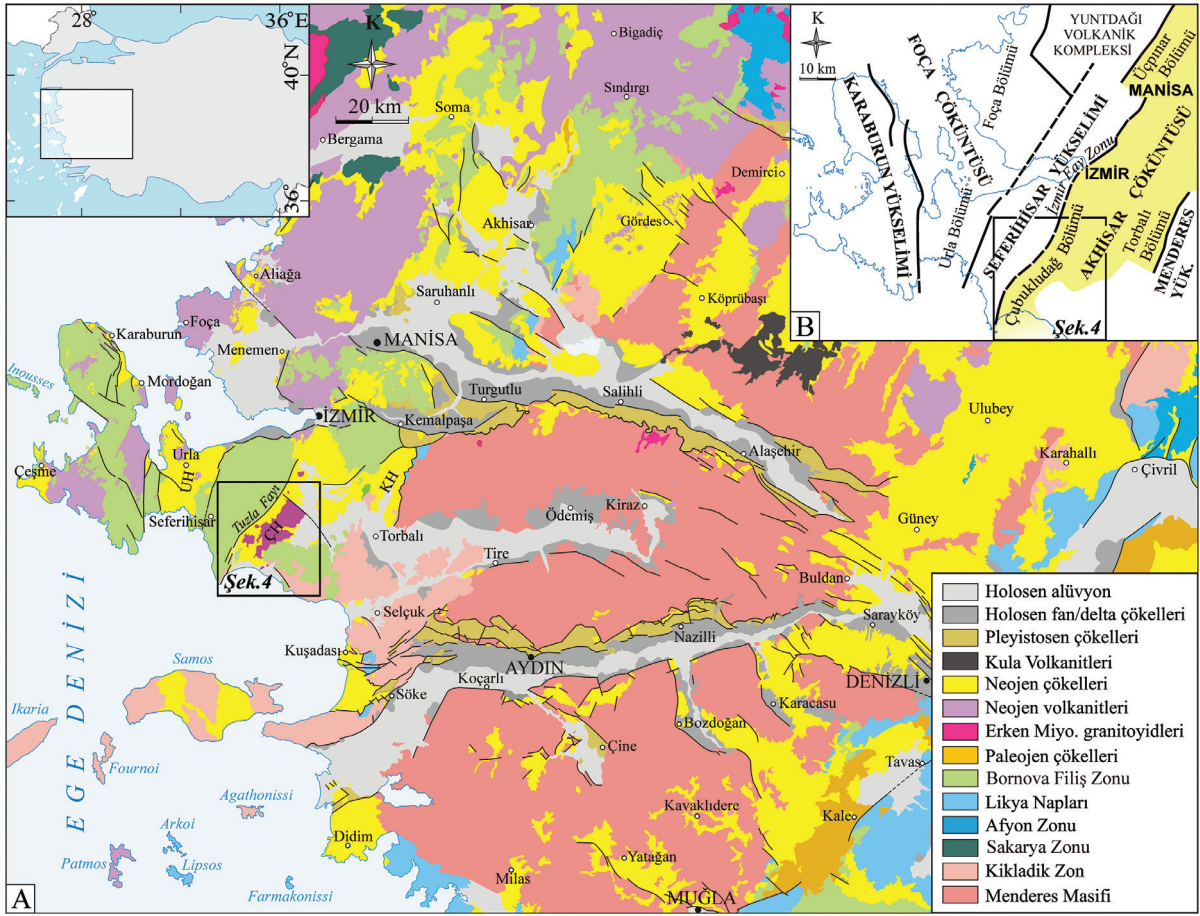
Şekil 1. A) Çubukludağ havzasının bölgesel jeolojik konumu ve B) Akhisar Çöküntüsü (Kaya, 1979) içindeki yeri. ÇH: Çubukludağ havzası, KH: Kocaçay havzası, UH: Urla havzası.
