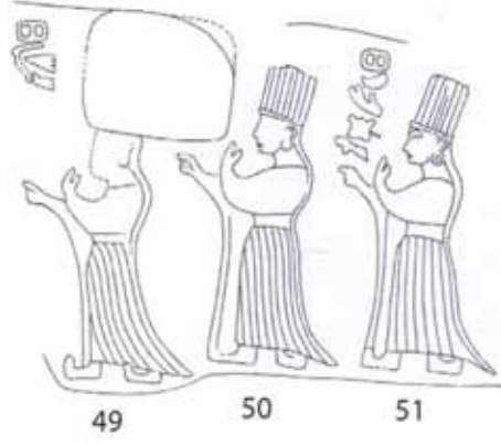
Res. 1: 50 nolu rölyef tanrıça İřhara ile irtibatlandırılmaktadır. Çizim için bkz. Seeher 2011: Res. 76: 74.
