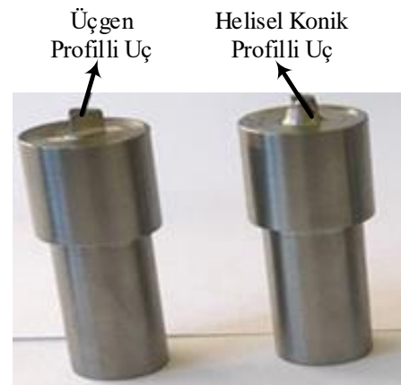
Şekil 2. SKK işleminde kullanılan farklı geometrilerdeki uçlar
