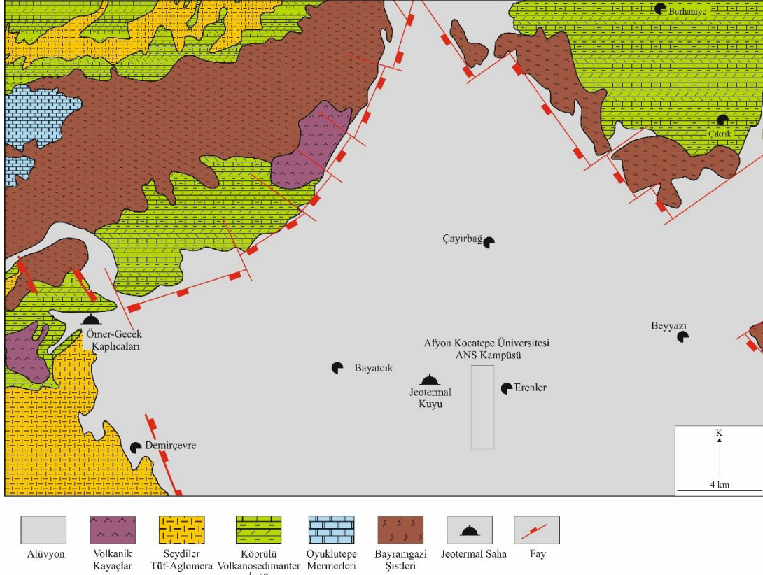
Şekil 1. İnceleme alanının jeoloji haritası (Ulutürk, 2009; Yıldız vd., 2012'den değiştirilerek alınmıştır).
