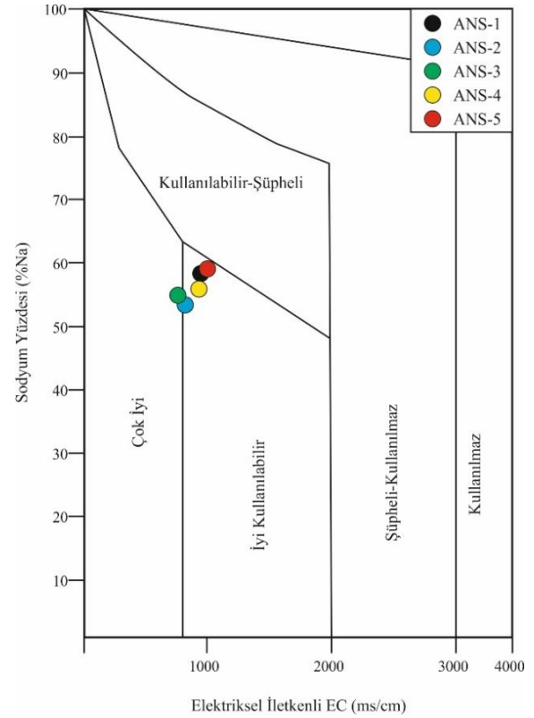
Şekil 7. Wilcox diyagramı.
