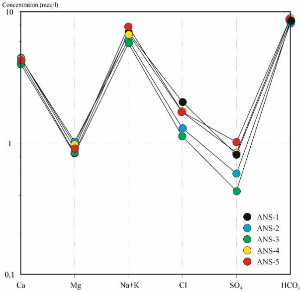
Şekil 3. Schoeller diyagramı.
