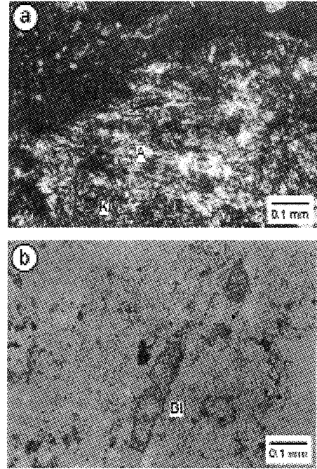
Şekil 3. Bozuşmuş volkanik kayaların mikrofotografaları, a) Kaolinit kitap demetleri ve prizmatik alünitler (Canabdal yöresi, GT-14, çift nikol; K=Kaolinit, A=Alünit), b) Kalsedonik matriks içinde özşekilli baritlerin dizilişi (Kiremitli yöresi, YK-15, tek nikol, Bt=Barit).
