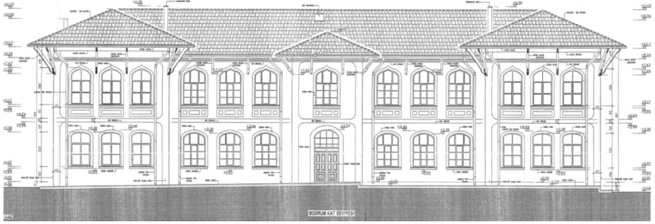
Çiz. 4: Güney Cephe Görünüşü. (Rölöve projeleri Birikim Mimarlık tarafından hazırlanmış olup; projelere Orhan Gazi İlkokulu arşivinden ulaşılmıştır.)
