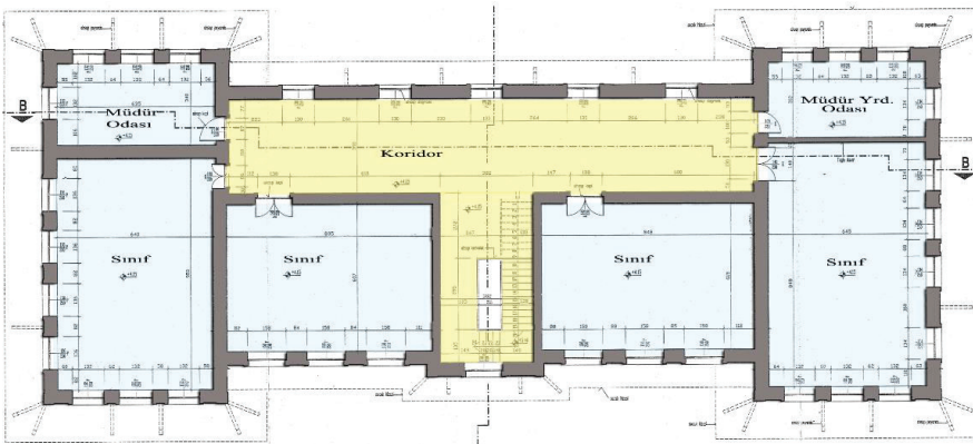
Çiz. 3: Bodrum, Zemin ve Birinci Kat Planları. (Rölöve projeleri Birikim Mimarlık tarafından hazırlanmış olup; kat planları yazarlar tarafından sadeleştirilerek renklendirilmiştir. Projelere Orhan Gazi İlkokulu Arşivi'nden ulaşılmıştır.)
