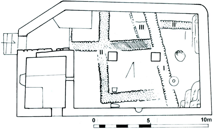
Çizim 2 - Kale Camii planı ve altındaki erken minari kalıntıları
