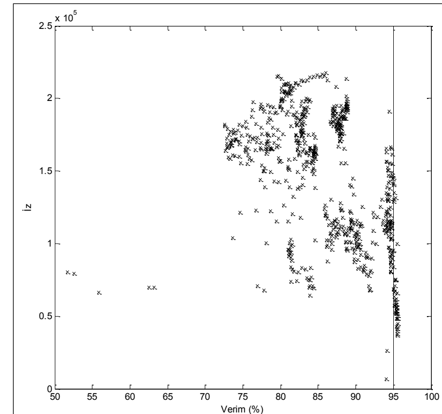
Şekil 5b. Kaynak Matrisi İzinin Verim ile Değişimi
