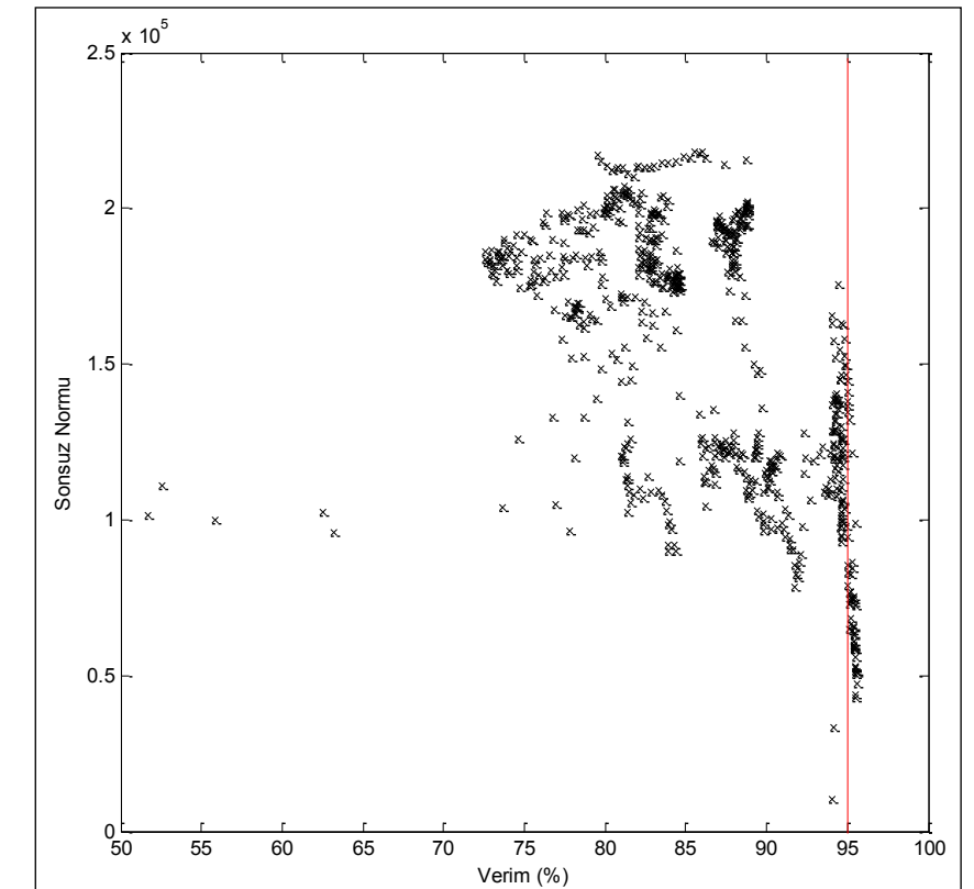
Şekil 3b. Kaynak Matrisin Sonsuz Normunun Verim ile Değişimi
