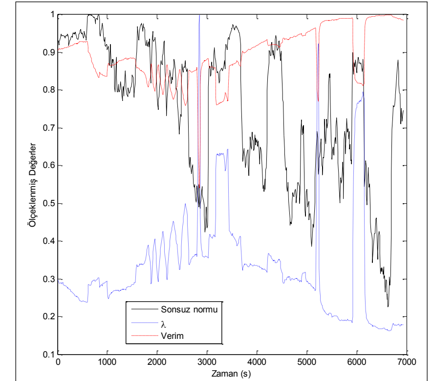
Şekil 3a. Görüntü Kaynak Matrisinin Sonsuz Normu ile Baca Gazı Analiz Cihazından Alınan Verim ve Hava Fazlalık Katsayısı Dataları
