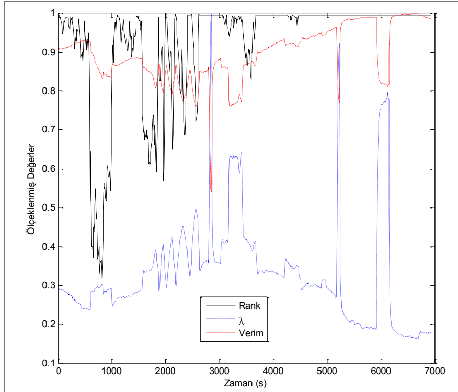
Şekil 4a. Görüntü Kaynak Matrisinin Rankı ile Baca Gazı Analiz Cihazından Alınan Verim ve Hava Fazlalık Katsayısı Dataları
