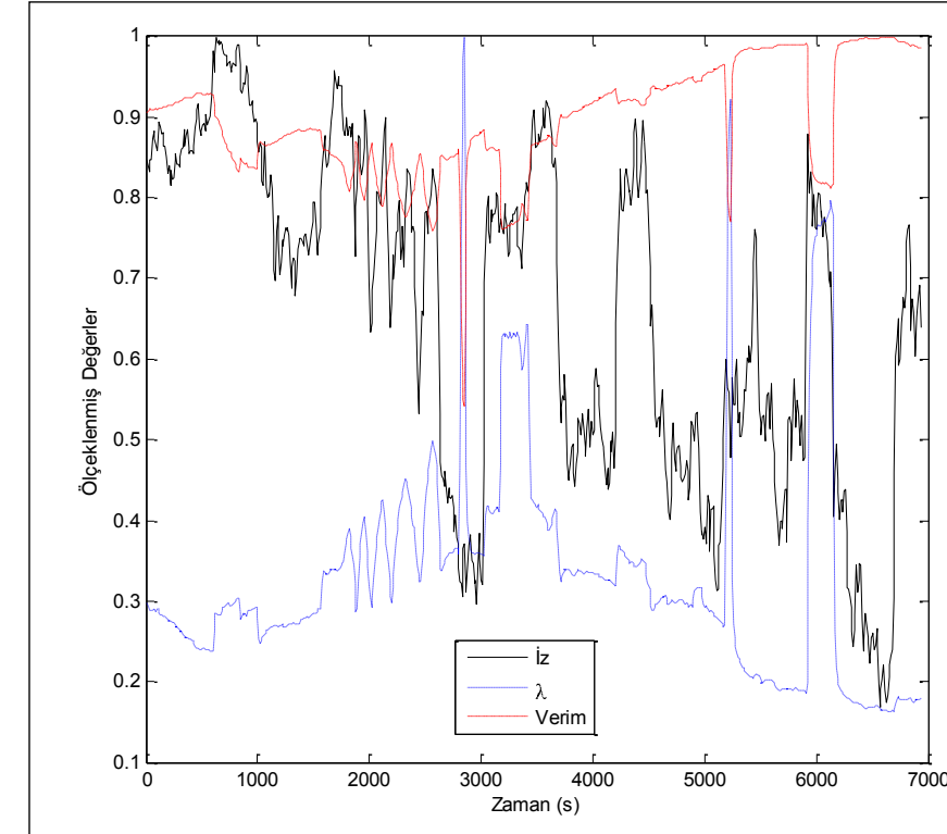
Şekil 5a. Görüntü Kaynak Matrisinin İzi ile Baca Gazı Analiz Cihazından Alınan Verim ve Hava Fazlalık Katsayısı Dataları
