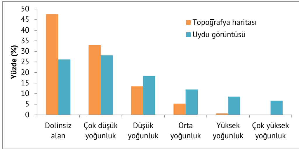
Őekil 3. Topoęrafya ve uydud grntlerine gre alıřma alanındaki dolin yoęunluk sınıflarının oranları.
