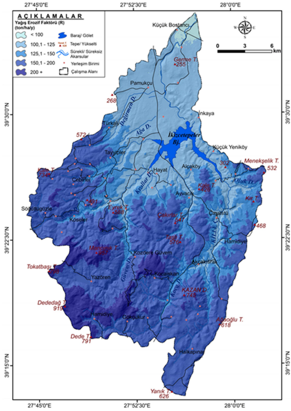
Şekil 3: Yağış (R) faktörü haritası / Figure 3: Map of rainfall (R) factor
