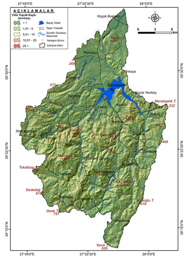
Şekil 7: Erozyon risk sınıfları ve toprak kaybı haritası / Figure 7: Erosion risk classes and soil loss map
