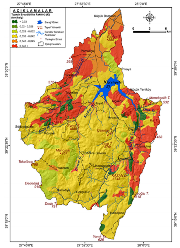
Şekil 4: Toprak (K) faktörü haritası / Figure 4: Map of soil (K) factor
