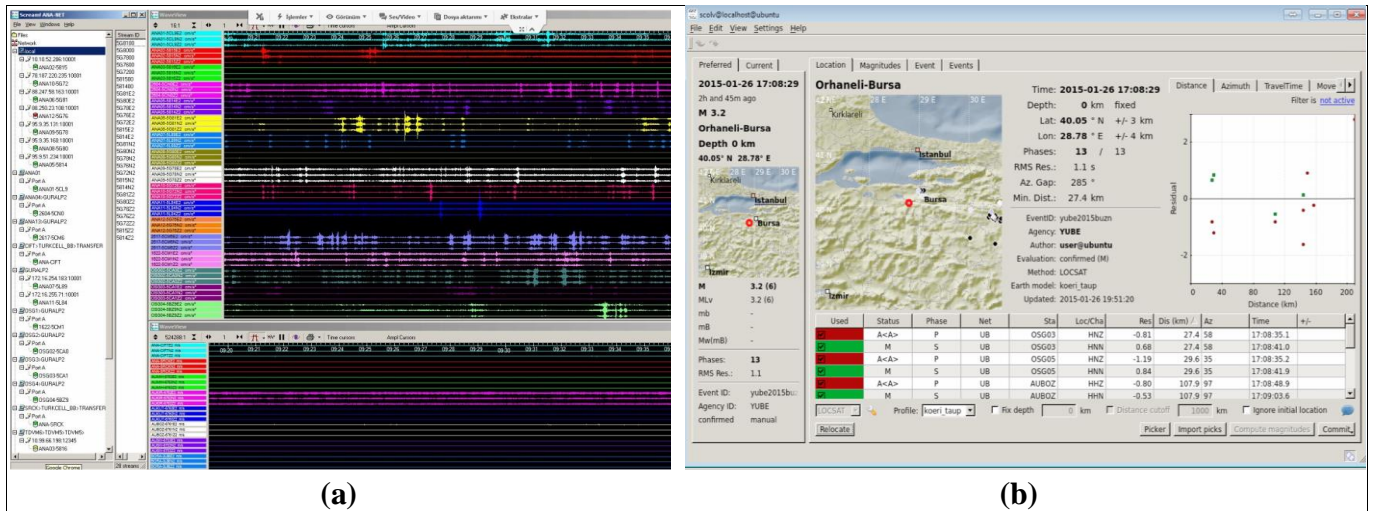
Şekil 6. (a) AnaNet Sismik ağı istasyon kontrol ve veri izleme ekran görüntüsü (Scream ile) (b) AnaNet Sismik ağı istasyon durum bilgisi ve deprem çözümlene ekran görüntüleri (SeisComp3 ile)
