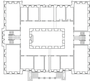
Çizim 19. Kongre Mürzesi Zemin Kat Planı K
