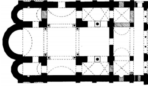
Görsel 4 Edirne Ayasofya Cami planı (Günözü,2014)
