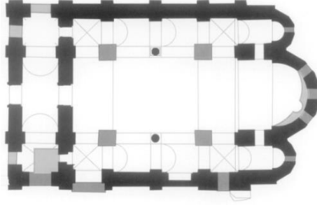
Görsel 14 Kırklareli Ayasofya Cami Planı (Çavdar, 2014:12)
