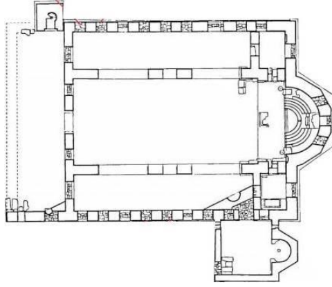
Görsel 12 İznik Ayasofya Cami Planı (Ermiş,2012)
