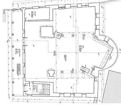
Görsel 18 Zonguldak Ayasofya Cami Planı (Karabük K.V.K., 2021).
