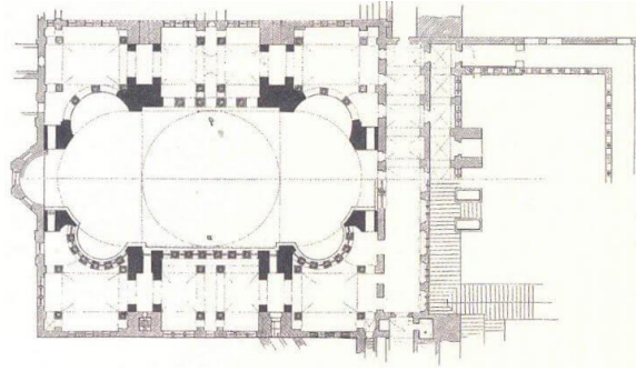
Görsel 8 İstanbul Büyük Ayasofya Cami Planı
