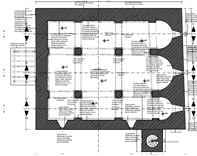
Görsel 2 Bitlis Ayasofya Cami Planı (Bitlis V.B.M., 2021)
