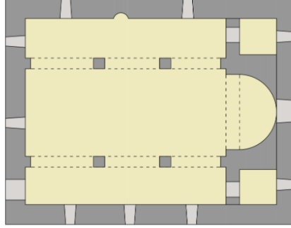
Görsel 6 Gümüşhane Ayasofya Cami Planı
