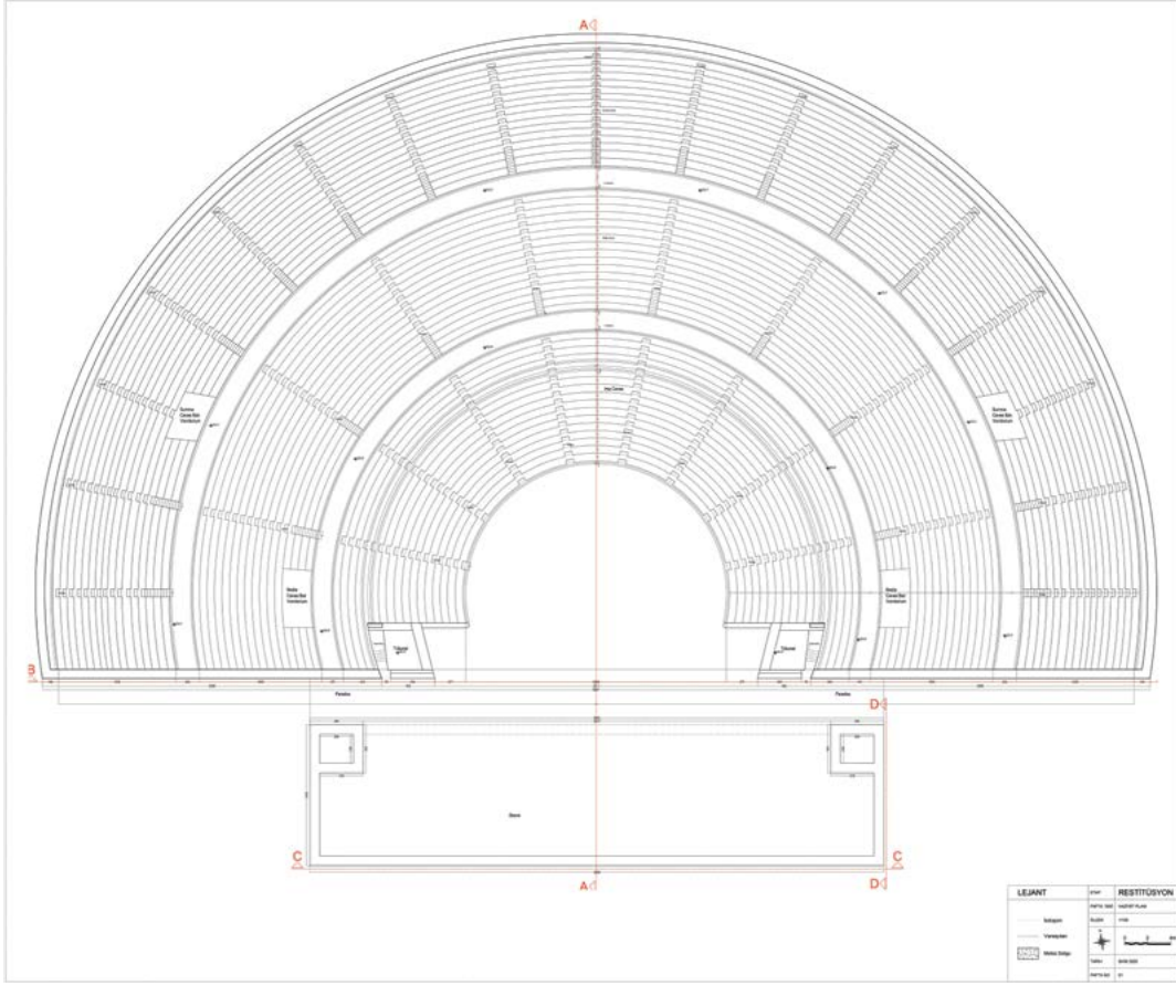
Fig. 3. Tiyatronun güncel planı
