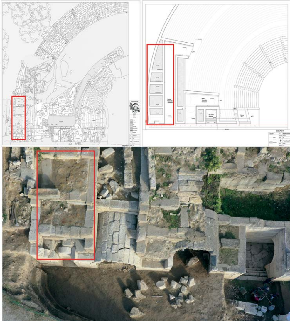
Fig. 4. Tonozlar üzerindeki basamakları destekleyen dolgu alanları
