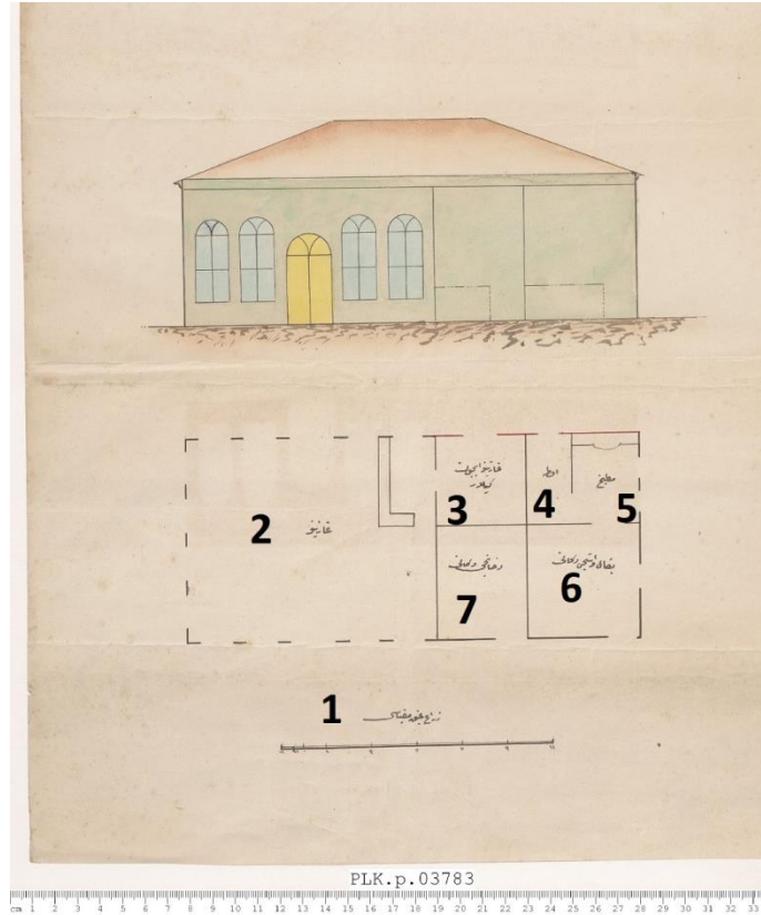
Resim 6. 1. Zirâ'-ı atik mikyâsı, 2. Gazino, 3 Gazino için kiler, 4. Oda, 5. Mutfak, 6. Bakkal ve aşçı dükkânı, 7. Duhancı dükkânı, (BOA., PLK.p., Dosya no: 3783).
