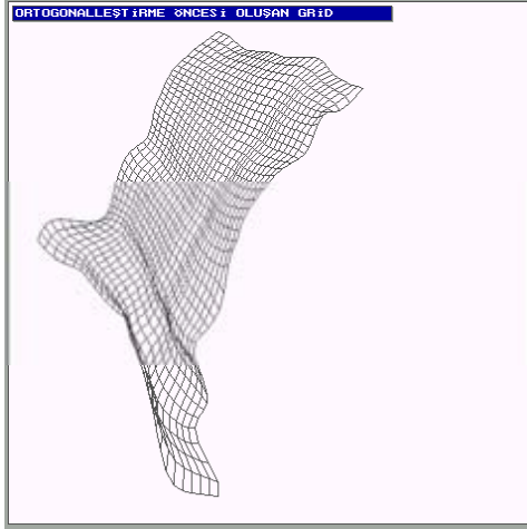
Şekil 15. Gökpınar test modelinin ortogonalleştirme öncesi oluşturulan ağ yapısı
