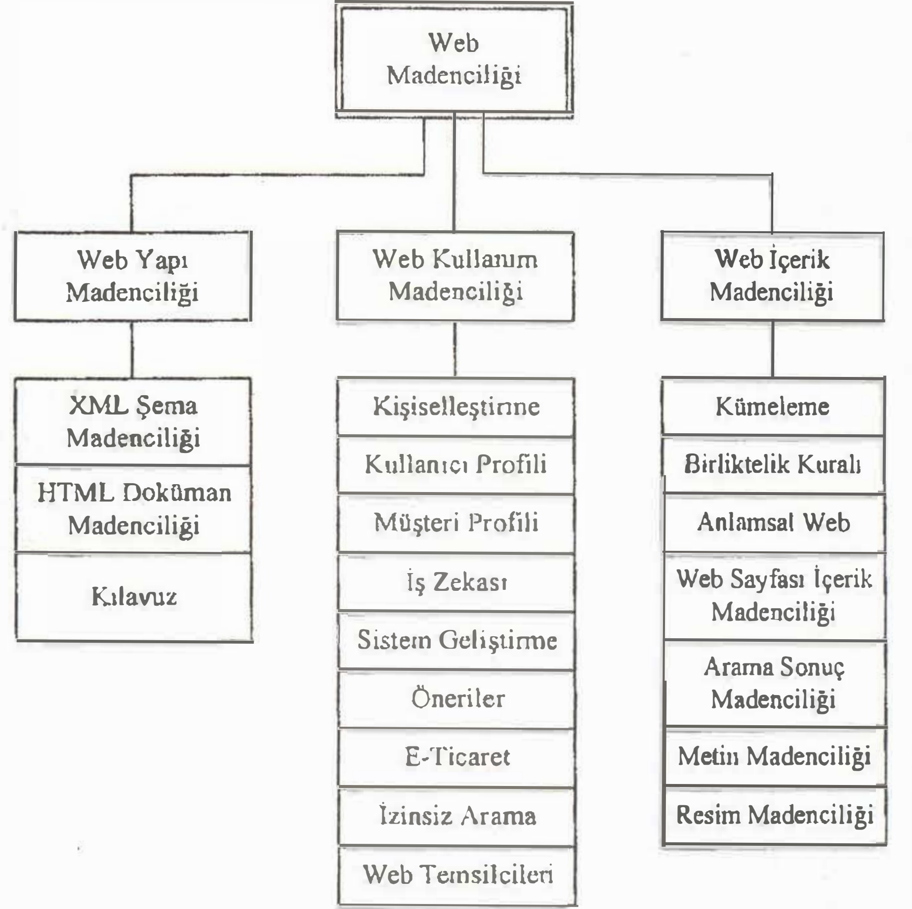
Şekil 1. Web Madenciliğinin Sınıflandırılması [8]
