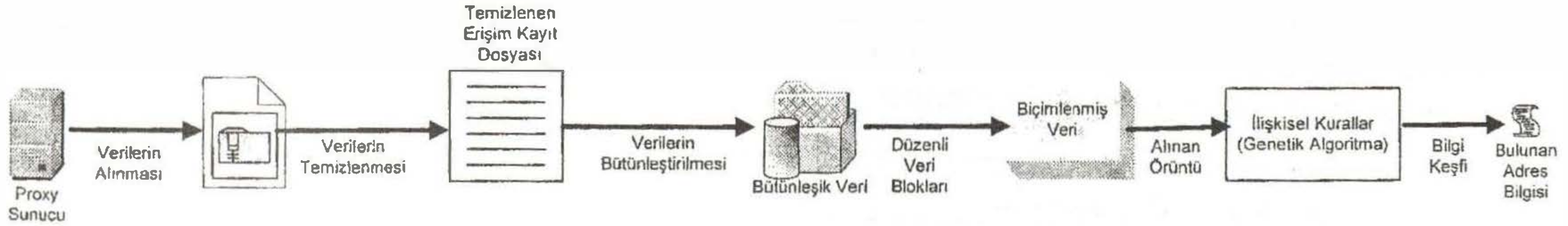
Şekil 2. Web Kullanım Madenciliği Mimarisi
