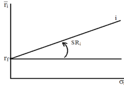
Şekil 2. Sharpe Endeksi
