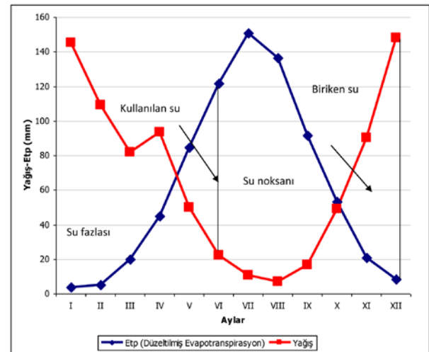
Şekil 2. Eğirdir'de Thornthwaite metoduna göre su bilançosu grafiği
