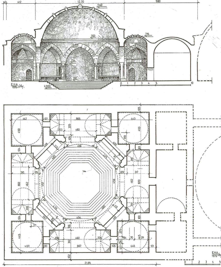
Çizim 6: Veli Bey Kaplıcası restitüsyonu (Çizim: A. Yüksel, 1976)
