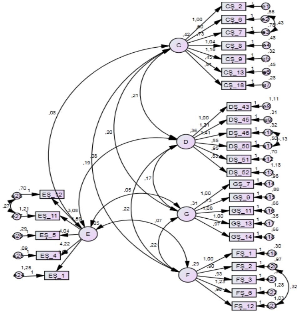
Diyagram 1. FŞTÖ'nün Doğrulayıcı Faktör Analizinin Geçerliliği
