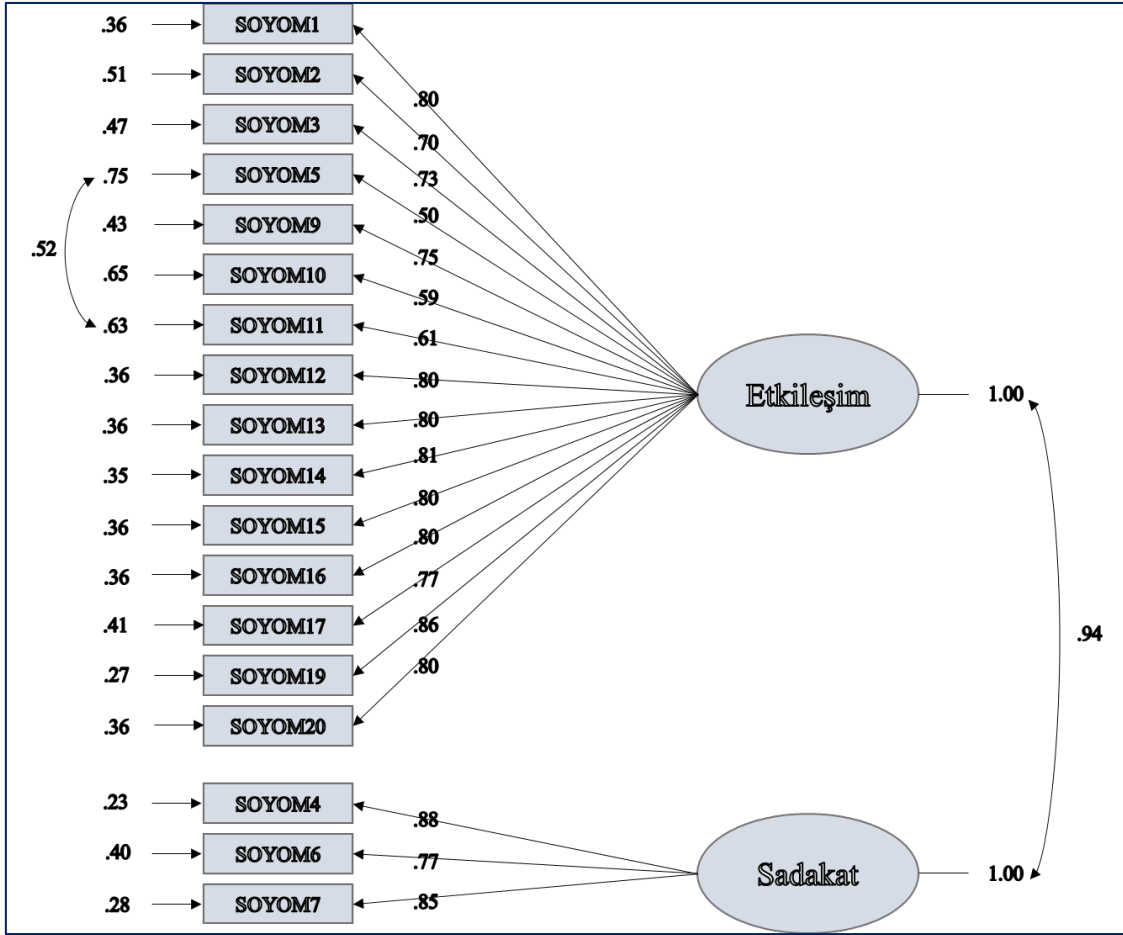
Şekil 1. ŞOYÖM Ölçeği Doğrulayıcı Faktör Analizi Sonrası Elde Edilen Model. \chi^2/sd = 1.92, p < .001, RMSEA = .10 . Not: SOYOM: Şiddet Olaylarının Yakın Öncülleri Mağdur Formu.
