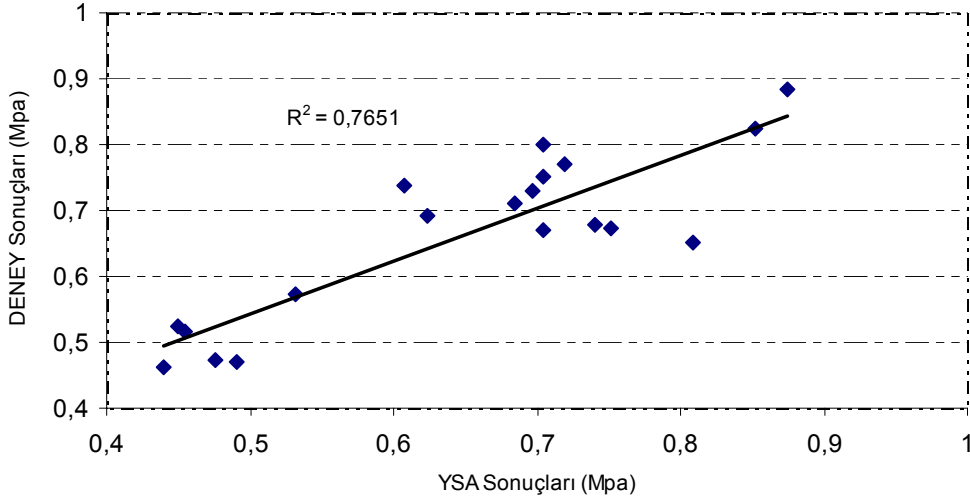
Şekil 8. Yarmada çekme dayanımı için YSA-DENEY ilişkisi (Test seti).
