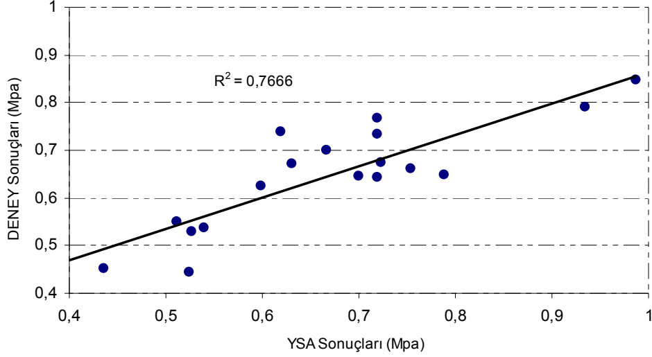
Şekil 7. Tek eksenli basınç dayanımı için YSA-DENEY ilişkisi (Test seti).
