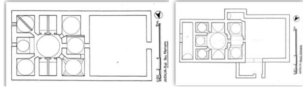
Fig. 43-44. Antalya Balibey ( Cumhuriyet ) ve Antalya Nazır Hamamı Planları (Yılmaz, 1997: 236-237)
