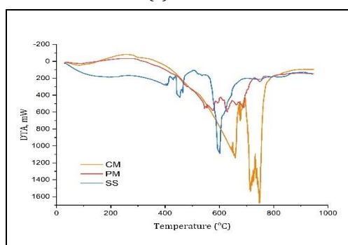
(b): DTA.
