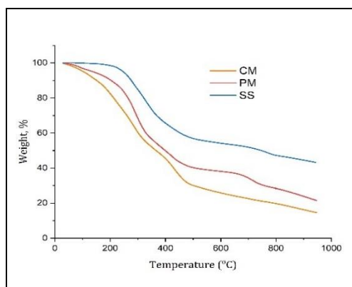
(a): TGA.
