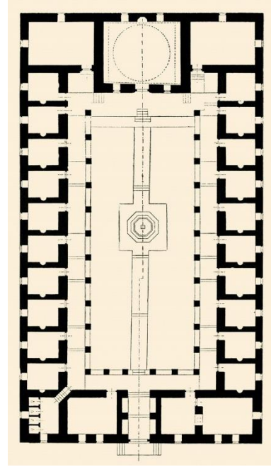
Resim 3. Yıldırım Bayezid Dârü'sşifası'nın planı (Sedat Çetintaş, Türk Mimari Anıtları , lv. 48/1)
