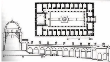
Resim 4. Yıldırım Darü'sşifasının Eğimli Yapısını Gösteren Çizim (Şener, 2014, s.45)
