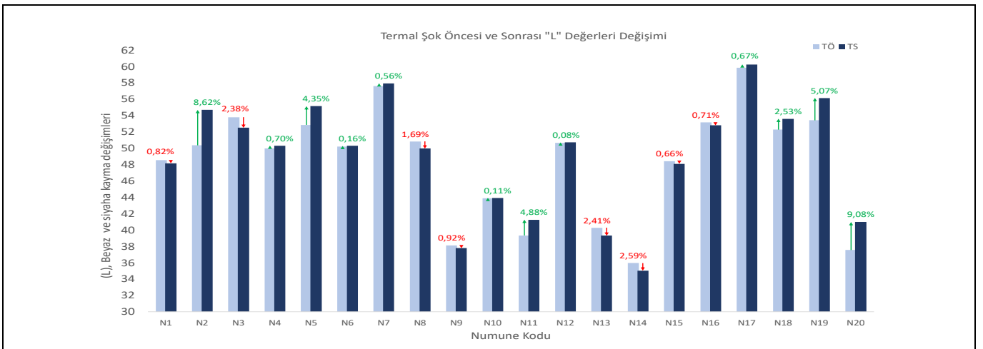
Şekil 10. Termal şok öncesi ve sonrası "L" değerleri değişimi. Figure 10. Change in "L" values before and after thermal shock.
