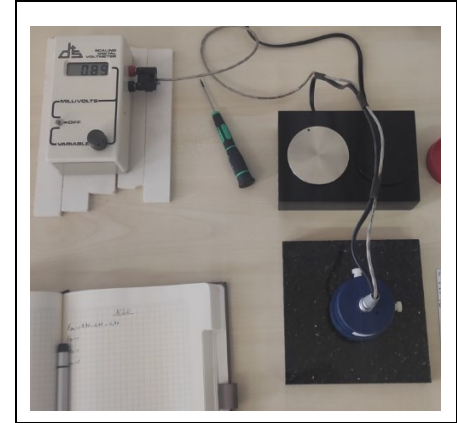
Şekil 6. Isıl Yayılımı Cihazı (termal emissometer) ile deney numunesinin \epsilon değerlerinin ölçülmesi.
