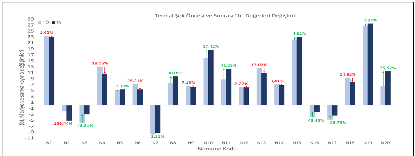
Şekil 12. Termal şok öncesi ve sonrası "b" değerleri değişimi. Figure 12. Change in "b" values before and after thermal shock.
