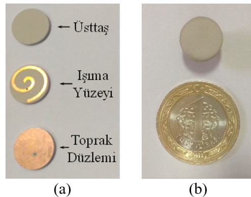
Şekil 11. Gerçeklenen ISM-bant AS-MİA'ya ait (a) katmanlı ve (b) üstten görüntüleri
