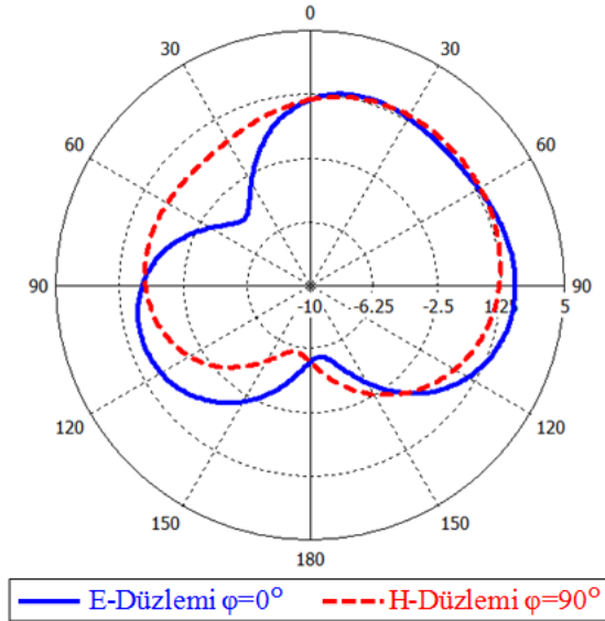
Şekil 5. Önerilen AS-MIA tasarımının ait 2.4GHz frekansındaki uzak-alan ışınma örüntüsü benzetim sonucu
