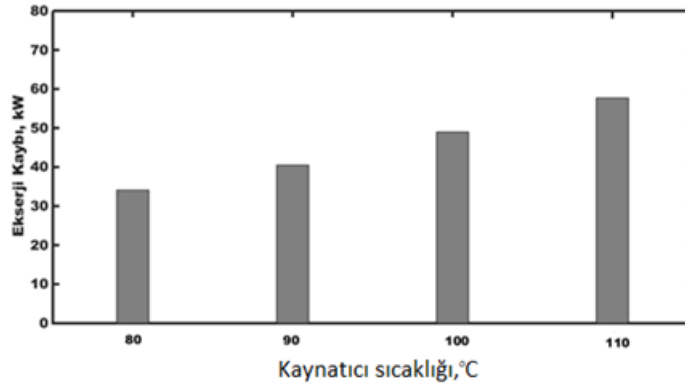
Şekil 6. LiBr-H 2 O akışkan çifti için kaynatıcı sıcaklığının toplam ekserji kaybına etkisi (T b =10°C, T abs =T y =40°C)
