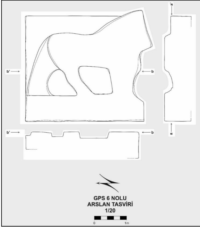
Çizim 1. Aslan Kabartma Taşlağının Çizimi (Çizen. Semih MUTLU).
