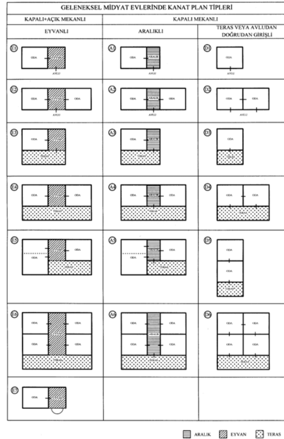
Şekil 7. Yapı kanat tipleri
